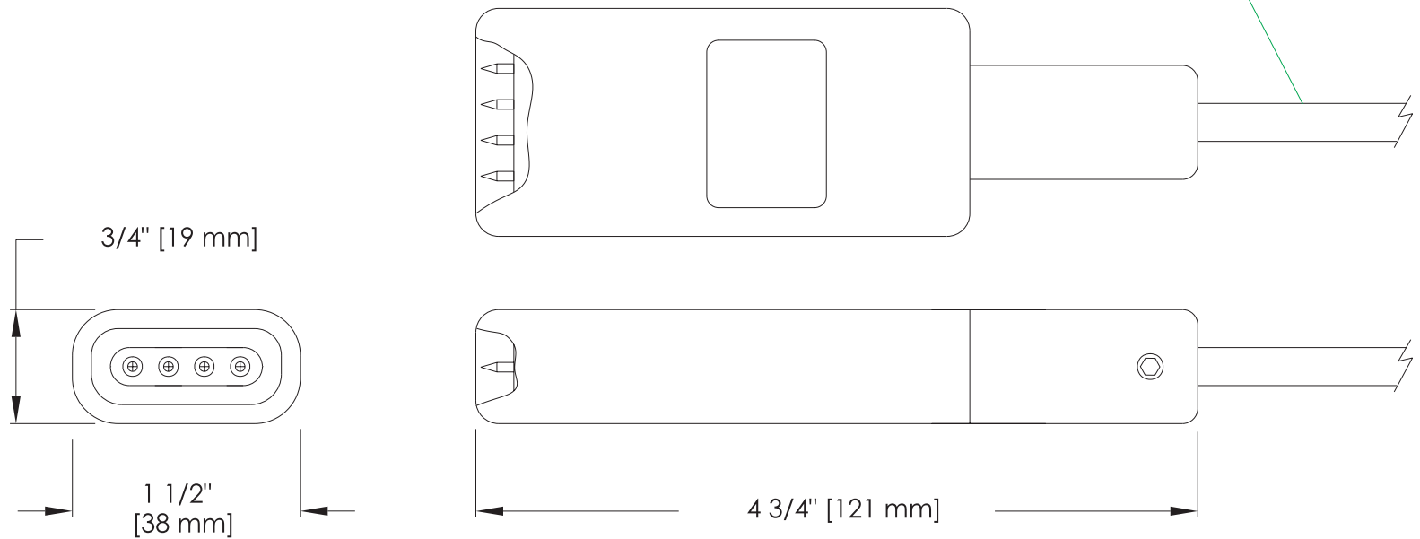
LINEAR PINNER
